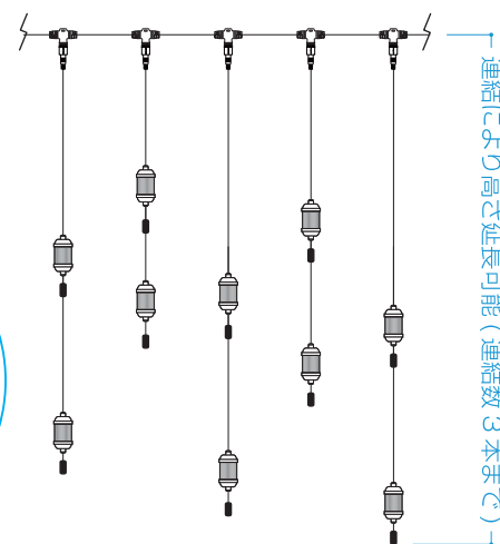
つららは1本づつ取り外しができ、連結ができます。 その為、長さ以外に高さを延長することも可能です。(連結可能数3本) ※つらら部分のみの販売は行っていません。
