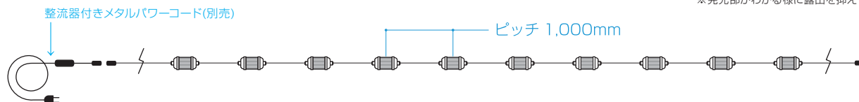
LEDフラッシュライト10 LED10球，ピッチ1,000mm LEDフラッシュライトタイプは全長9,000mm，ピッチ500mm，20球仕様での生産も可能です。
