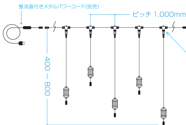
LEDフラッシュライトつらら 全体で5本のH400~800mmのつららで構成されています。
