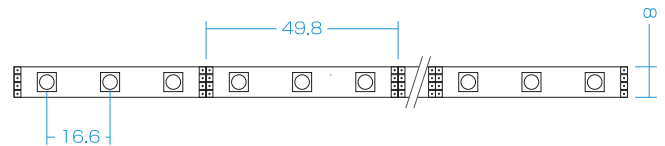
X-PANEL用 LEDモジュール(RGB)
