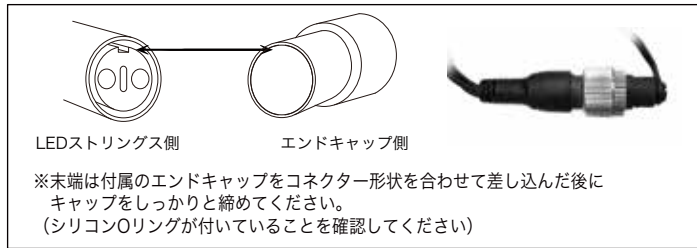
B 部拡大図
