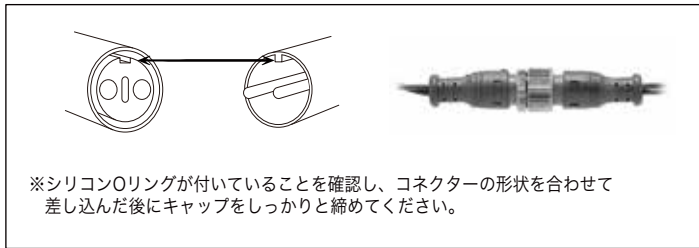
A 部拡大図
