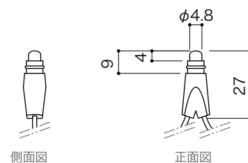
BULB拡大図
