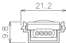
灯具+アルミライトレール 組立断面図
