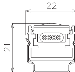
灯具+①+③ 組立断面図
