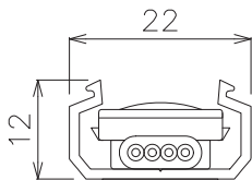
灯具+プラスチックモール 組立断面図
