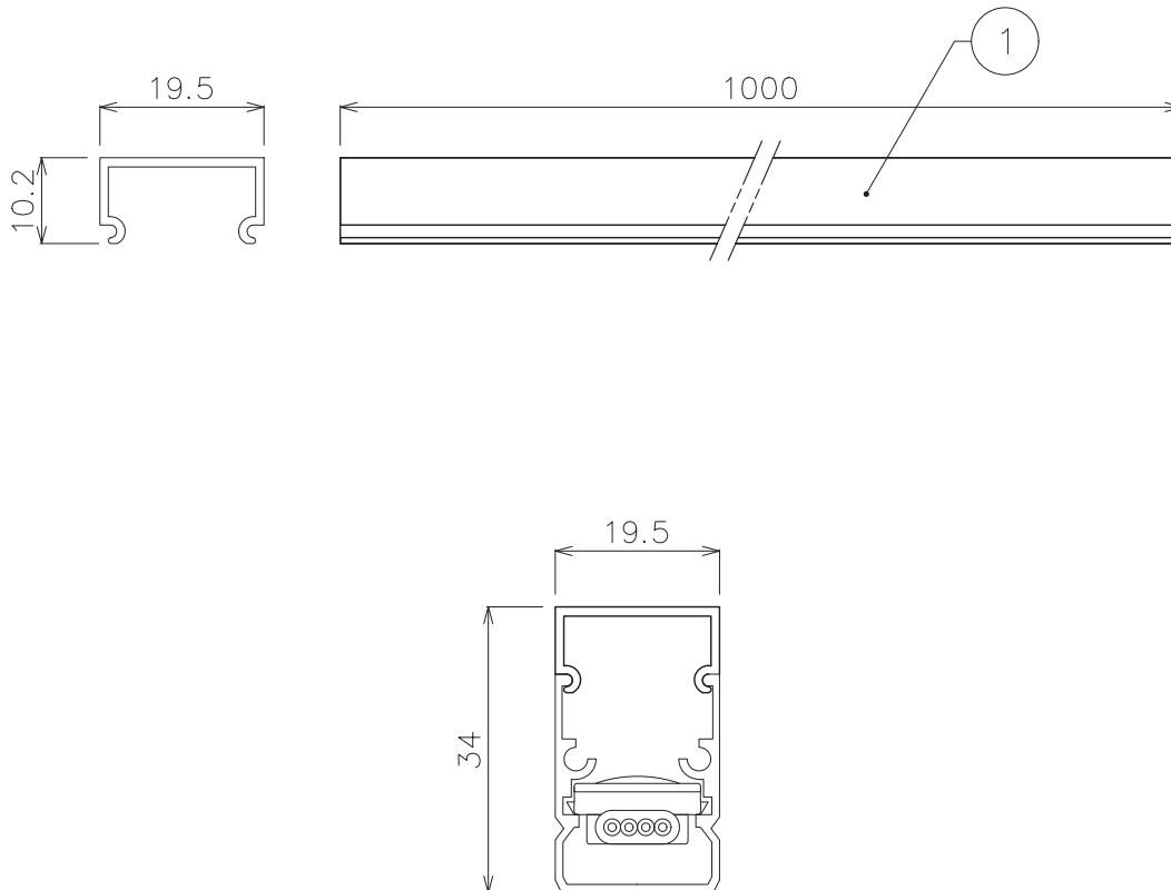
灯具+拡散カバー用アルミレール+拡散乳半カバー 組立断面図
