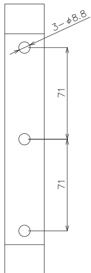
取付ベース穴位置
