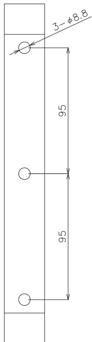
取付ベース穴位置
